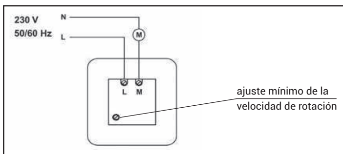
DIAGRAMA DE CABLEADO DEL CONTROLADOR
